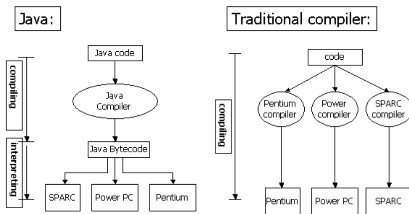
Slika 1.1 Usporedba izvršavanja Java programa s tradicionalnim postupkom prevodenja
